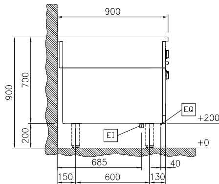
Zij aanzicht
